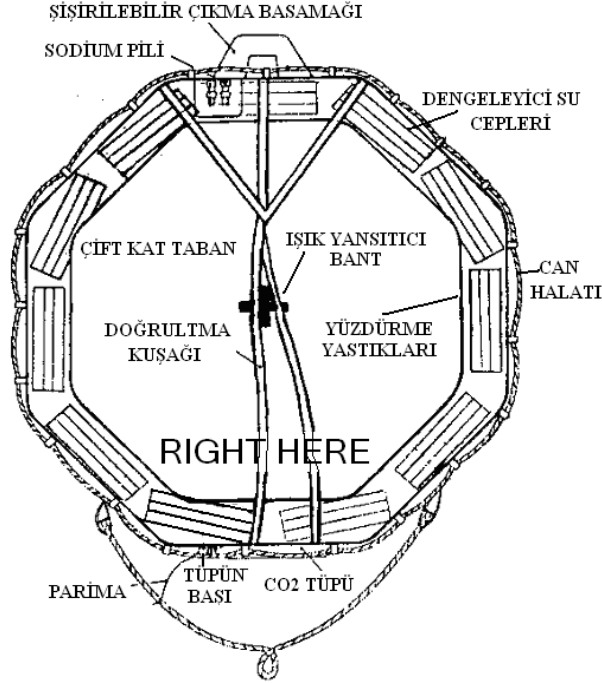
Şekil 1.19: Bir can salı taban yapısı
