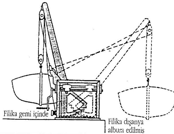
Şekil 1.7: Palangalı mataforalı can filikası indirme cihazı
