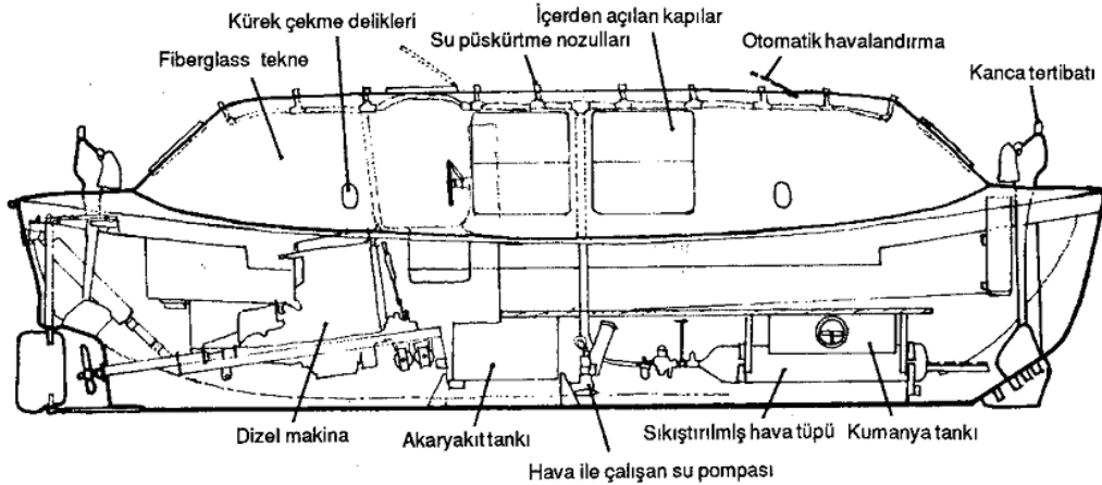
Şekil 1.2: Tam kapalı can filikası ve kısımları
