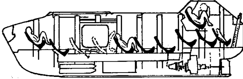
Şekil 1.14: Kızaklı serbest düşürmeli bir kapalı can filikasının kesiti
