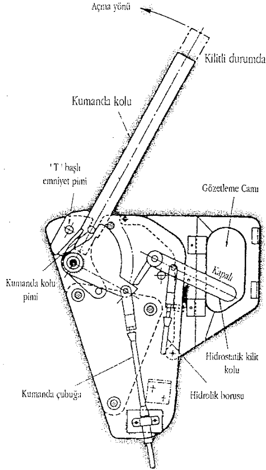
Şekil 1.13: Kapalı filika kanca açma tertibatı
