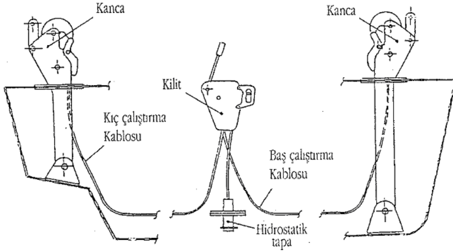
Şekil 1.12: Filika askı kancasını açma düzeneği
