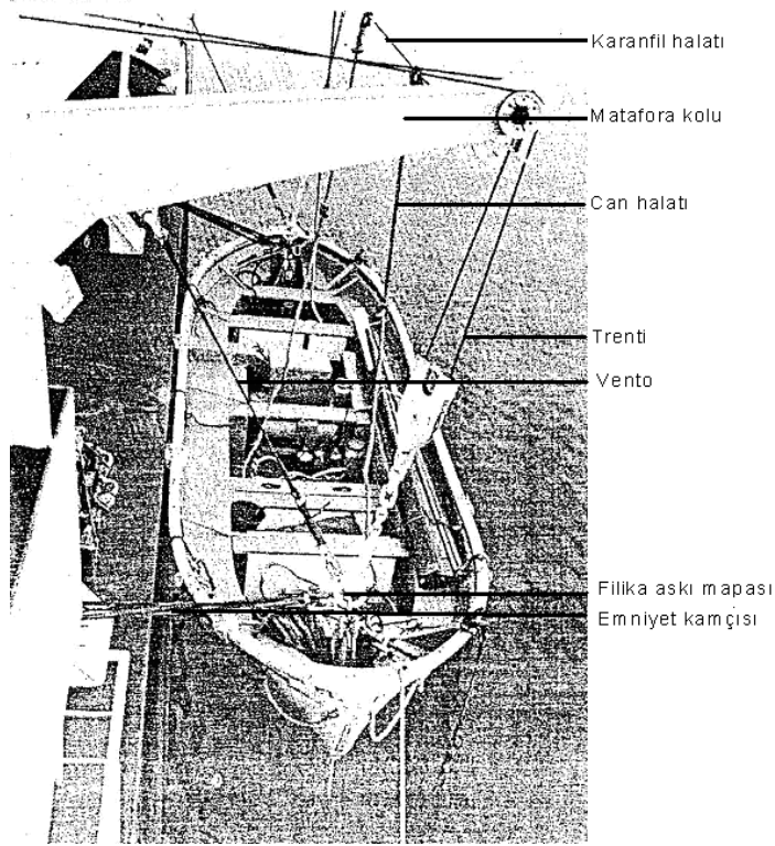
Şekil 1.9: Güverte hizasına indirilmiş bir açık tip filika
