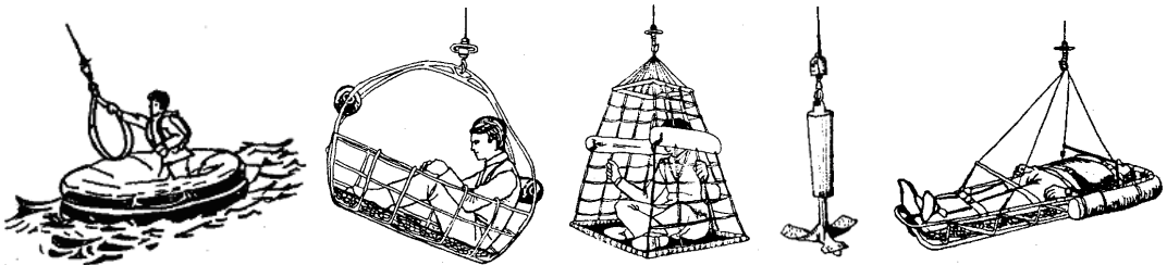
Şekil 2.10: Helikopter kazazede kurtarma teçhizatı
