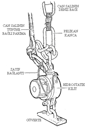
Şekil 1.6: Bir can salı emniyet kayışının bağlantısı
