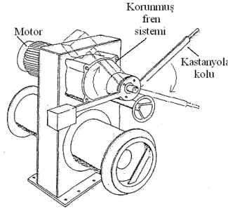
Şekil 1.10: Matafora motor ve fren aksamı
