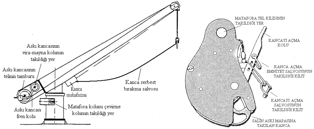
Şekil 1.17: Tek kollu matafora ve kancası
