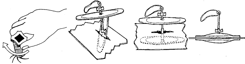
Şekil 1.21: Tapa ve kavrama ile saldaki hasarın onarımı
