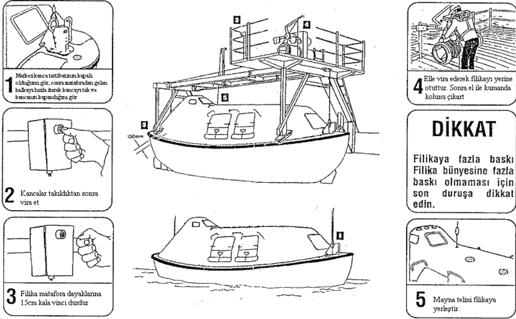
Şekil 1.18: Tam kapalı filikanın yerine alınması
