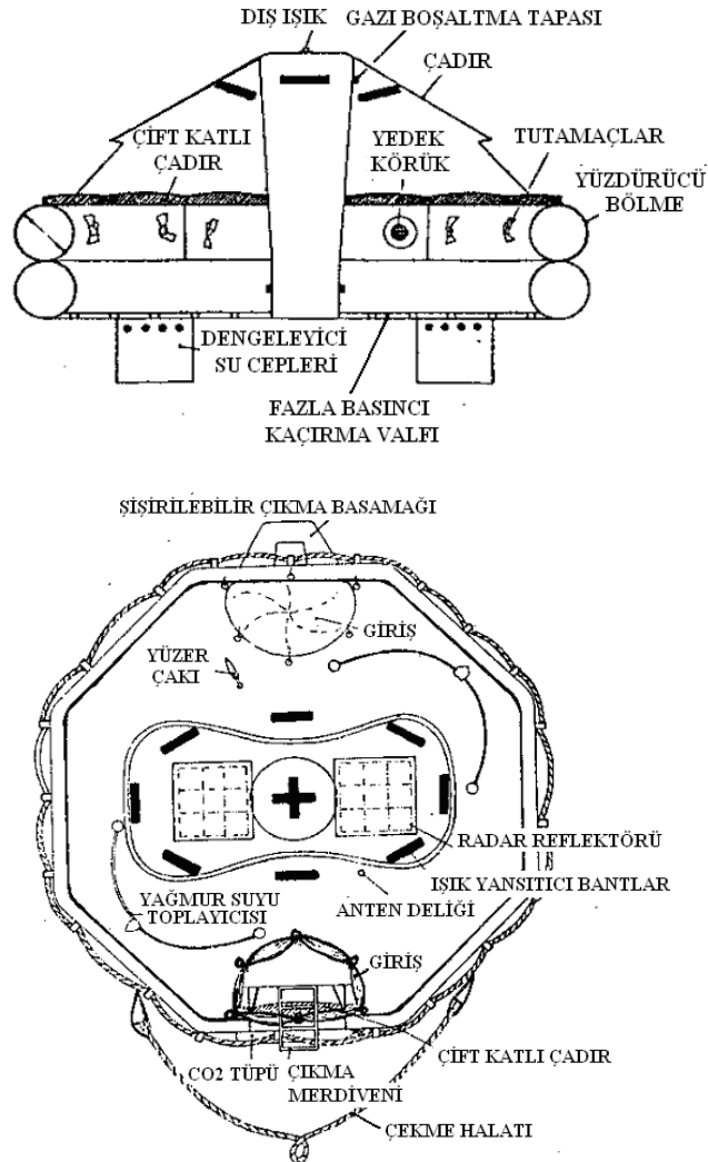
Şekil 1.3: Şişirilmiş bir can salı ve kısımları
