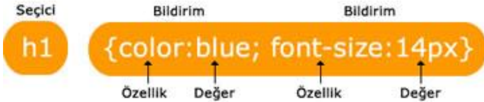
Şekil 1.1: CSS yapısı
