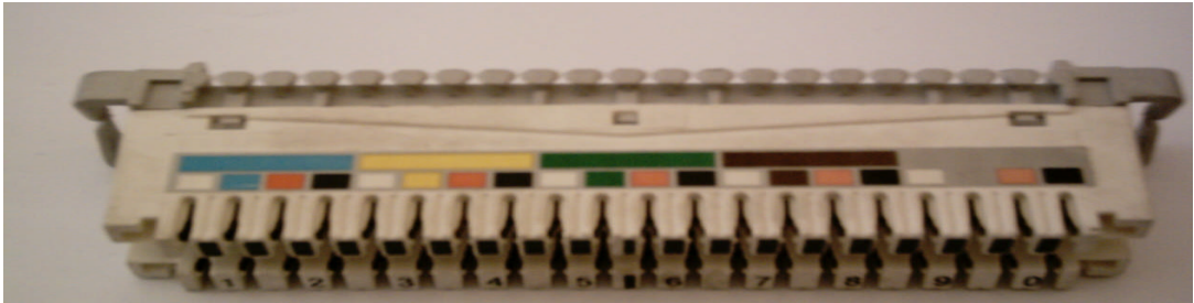
Resim 1.4: Prensibal ve yerel kabloların saha içinde bağlantı yapıldığı eleman (modül)
