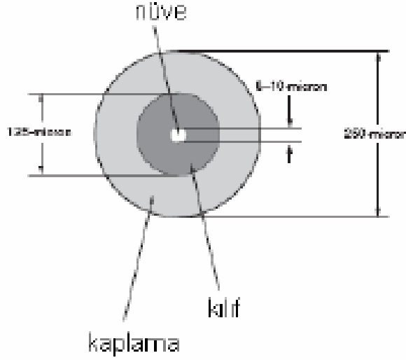
Şekil 3.3: Nüve/kılıf ölçüleri
