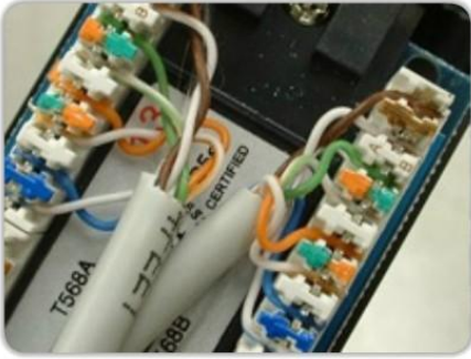
Bađlantı Panosunun Arka Tarafının Yakından Grnm
