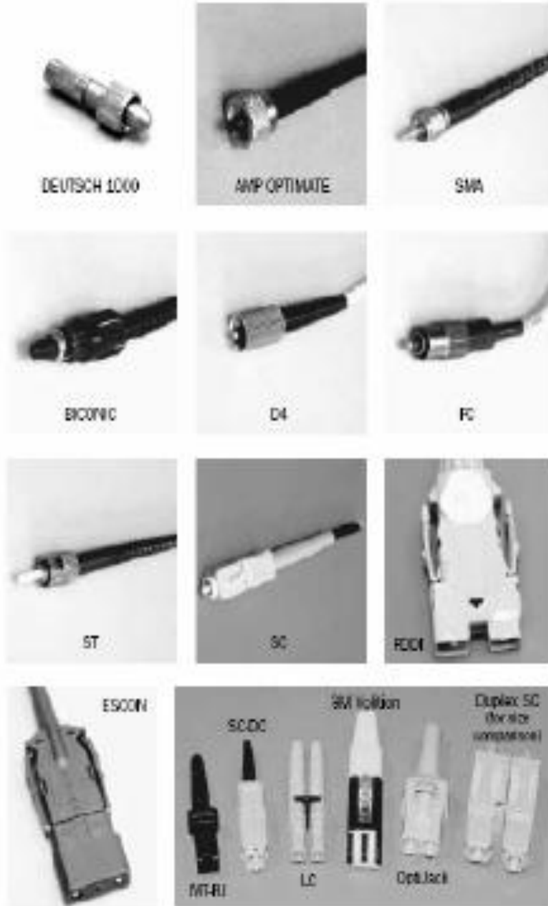
Şekil 3.5: Fiber optik kablolarda kullanılan konnektör tipleri
