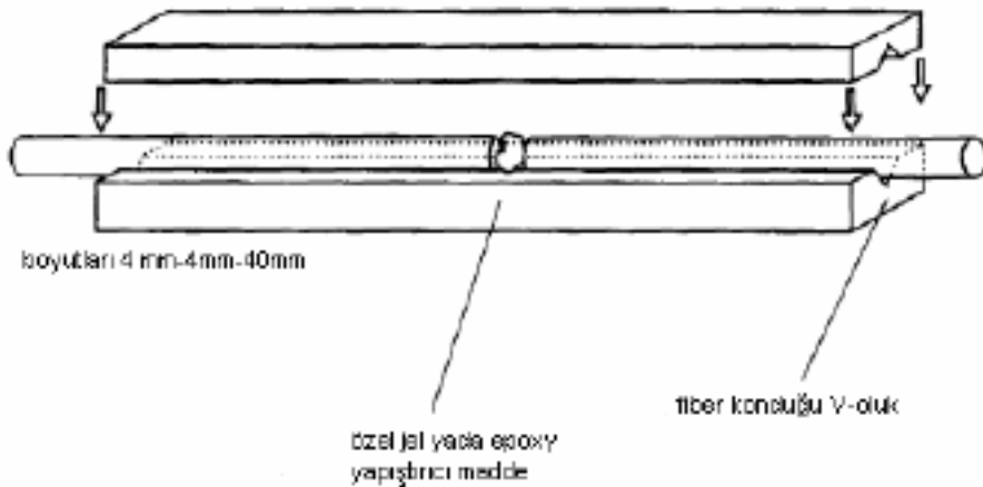
Şekil 3.27: Fiberlerin splice içinde eklenmesi
