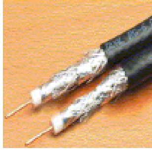
Şekil 2.1: Koaksiyel kablo
