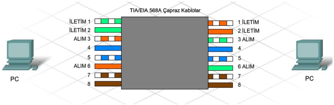
Şekil 2.13: Çapraz bağlantı
