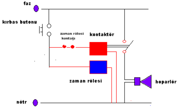
Şekil 2.13: Kır-bas sisteminin çalışma prensibi
