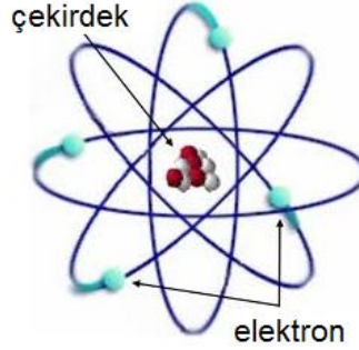
Resim 4.2: Atom modeli
