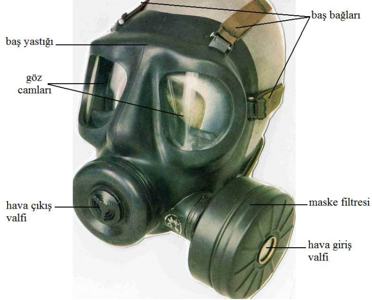
Resim 1.7: Gaz maskesi başlığı ve filtresi
