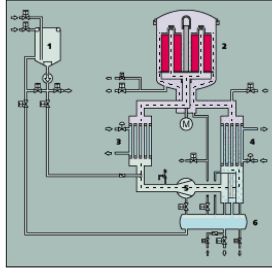
Şekil 2.1: Bobin iplik boyama makineleri
