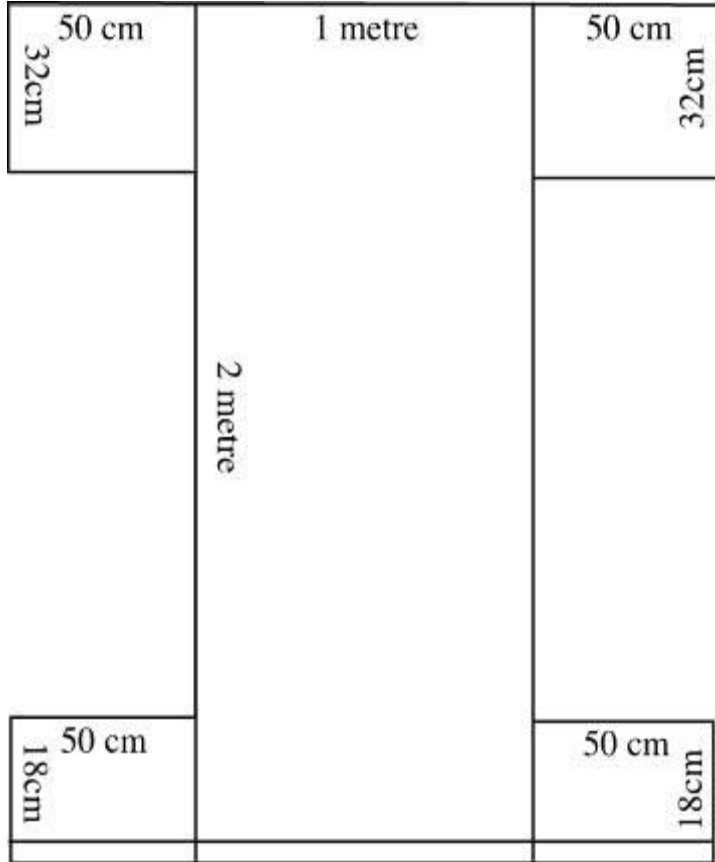
Şekil:1.1. yorgan hurcu kalıbı
