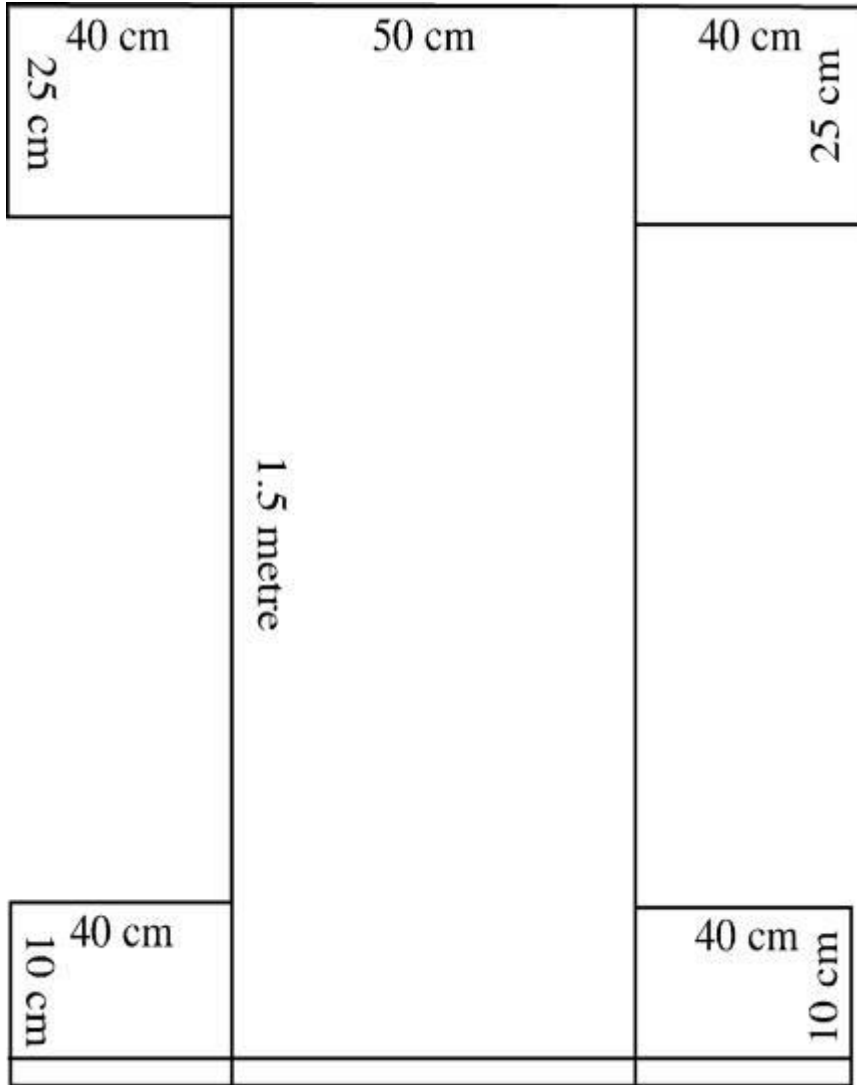
Şekil:1.2. Kazak Hurcu Kalıbı
