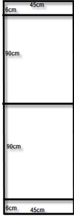
Şekil:1.4.Halı Hurcu Kalıbı
