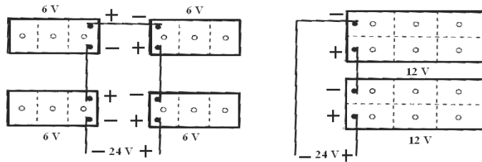
Şekil 4.2: Akümülatör bağlantıları
