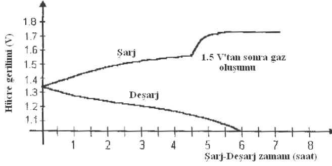
Şekil 4.5: NiCd akümülatörün şarj-deşarj grafikleri
