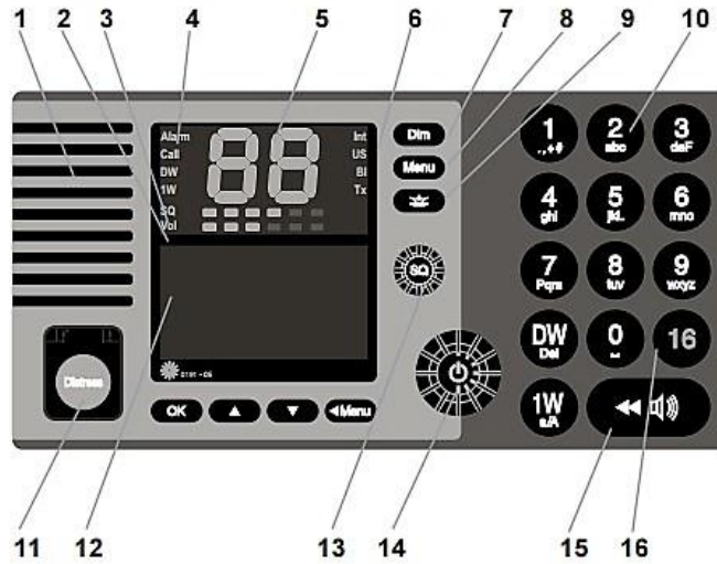
Şekil 1.2: VHF DSC cihazı
