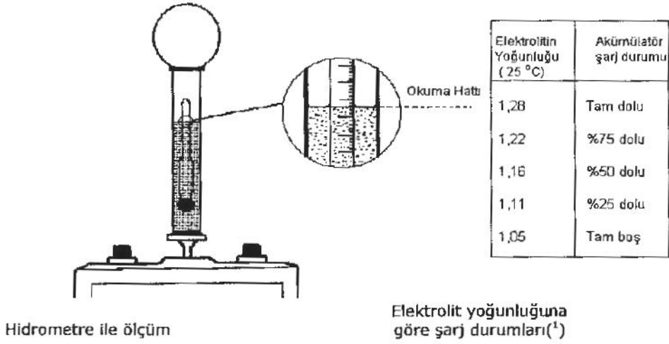
Şekil 4.4: Akü elektrolit yoğunluk ölçümü
