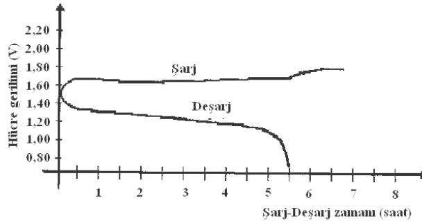
Şekil 4.6: NiFe akümülatörün şarj-deşarj grafikleri
