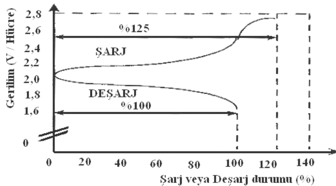
Şekil 4.3: Kurşunlu akümülatörün şarj - deşarj grafikleri
